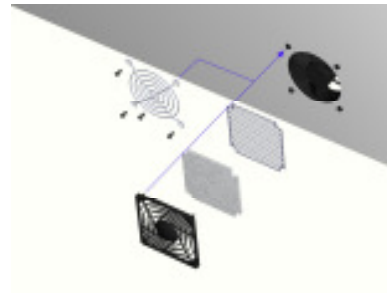
Metallschutzgitter
